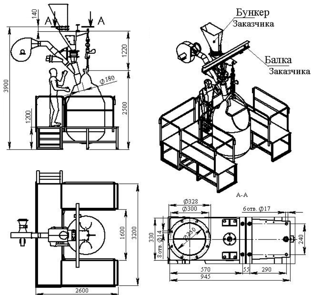
Рис. 1. Габаритно-установочные размеры.
